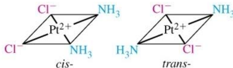
(b) izomeria cis i trans
