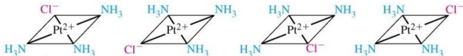
(a) brak izomerii
