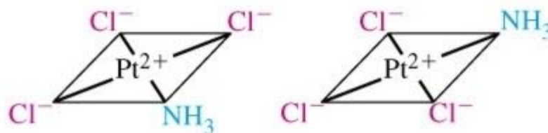
(c) brak izomerii
